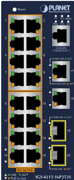
IGS-4215-16P2T2S
